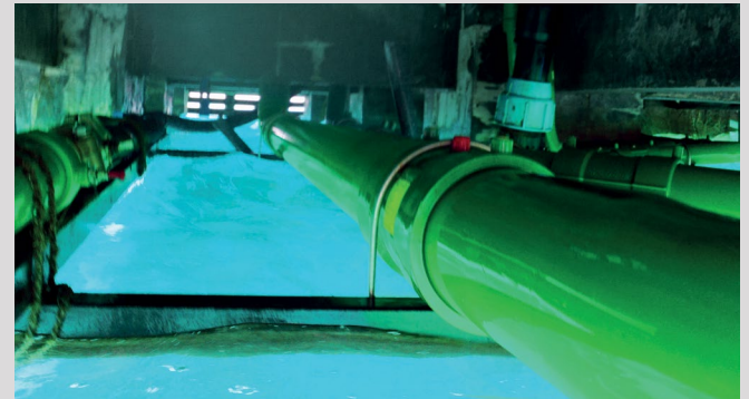
Birincil Jeneratör için Yakıt Dağıtım İskelesi, Maldivler
