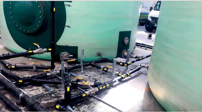
Instalaciones de producción de Adblue de Maxol – Ireland
